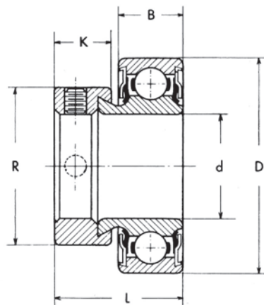
Cylindrical O. D. RA100
